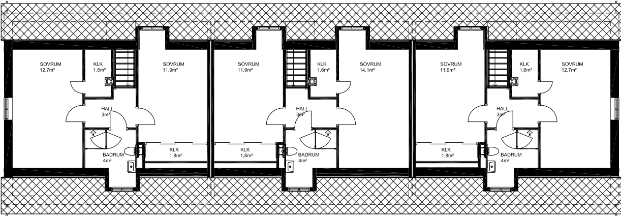
Våning 2
