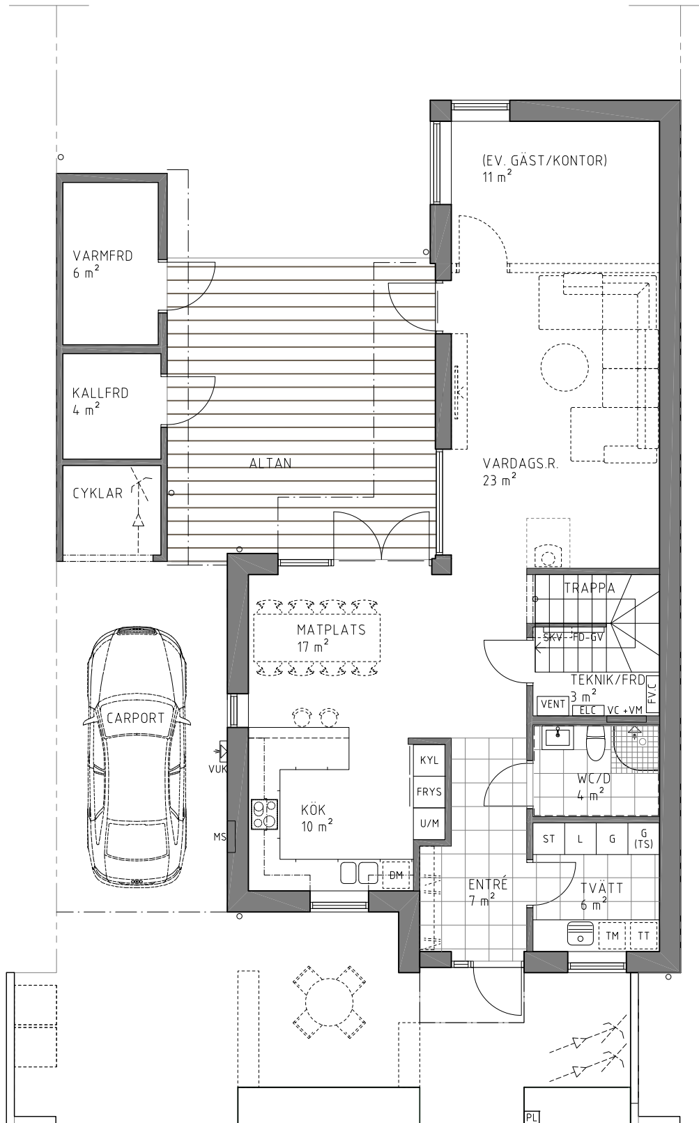
ENTRÉPLAN, PLAN 1
